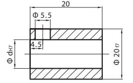
SK09 - RH Diğer delik çapları Ø10, 11, 12, 14, 15, 16, 18mm
