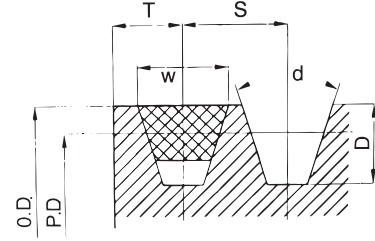
STANDART YIV ÖLÇÜLERİ
