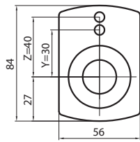
Sabitleme Pimi Pozisyonu Y ya da Z
