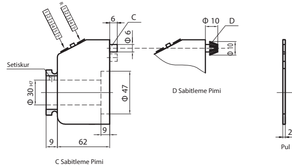
Sabitleme Pimi Pozisyonu Y ya da Z
