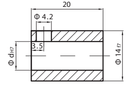
SK04 - RH Diğer delik çapları Ø6, 8, 10, 12mm
