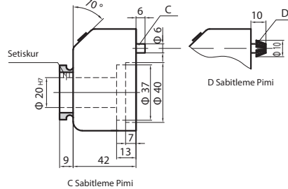
C Sabitleme Pimi
