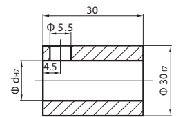
SK10 - RH Diğer delik çapları Ø20, 22, 24, 25, 26mm
