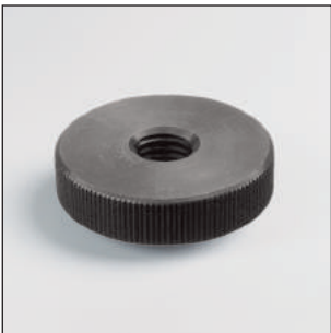
Dış çekilmiş, delikli. Fe: Çelik kalitesi 5, karartılmış. 376800120 numaralı malzeme DIN standartlarına uygun değildir.
