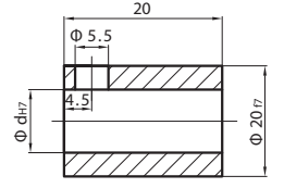
SK19 - RH Diğer delik çapları Ø10, 11, 12, 14, 15, 16, 18mm
