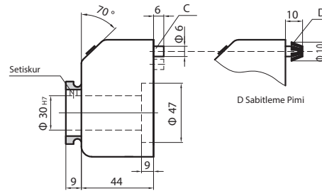
C Sabitleme Pimi
