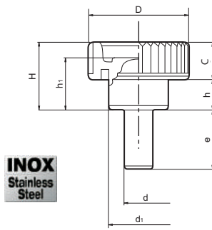
Paslanmaz-çelik cıvatalı (AISI 303). PA: Poliamid.
