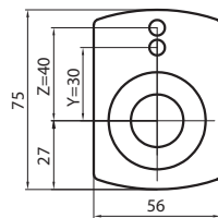
Sabitlenme Pimi Pozisyonu Y ya da Z
